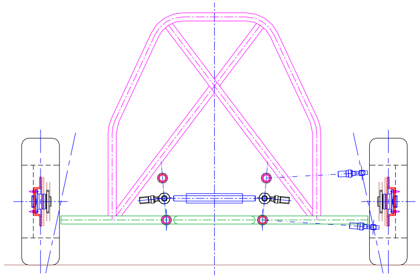
Рисунок 6.1. Проработка компоновки передней подвески.
